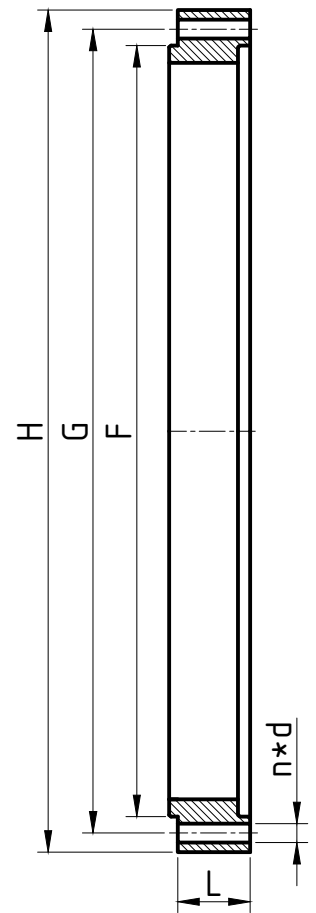
distantni prsten
