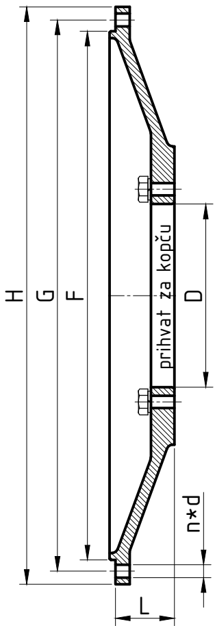
zvono tanjurasto
