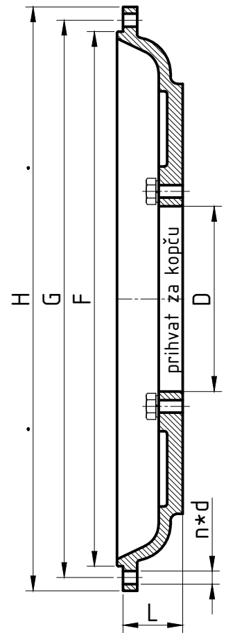
zvono konkavno
